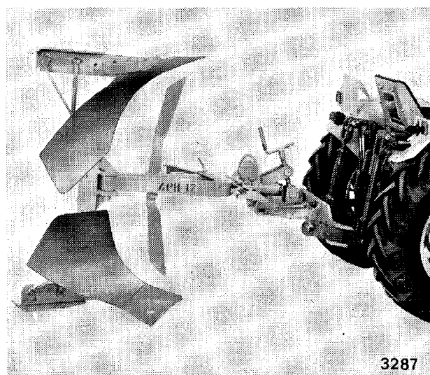
Aratro voltaorecchio a 180° modello « ZPH17 » (fig. 44).
