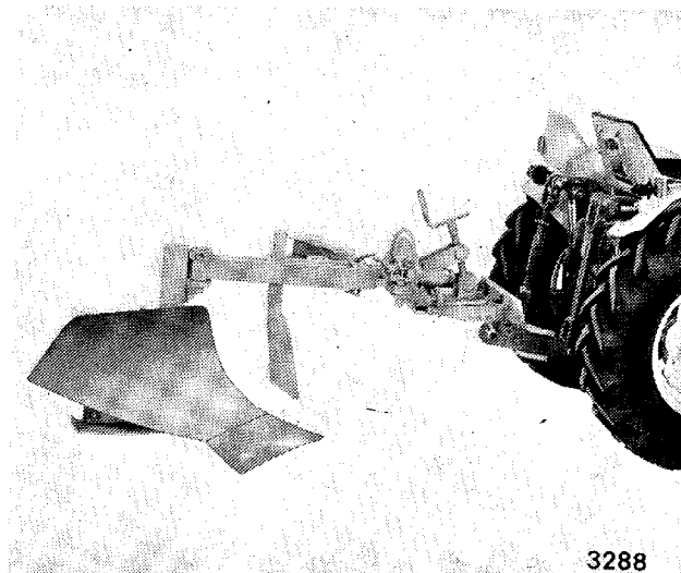
Aratro monovomere modello « MPH17 » (fig. 42).
