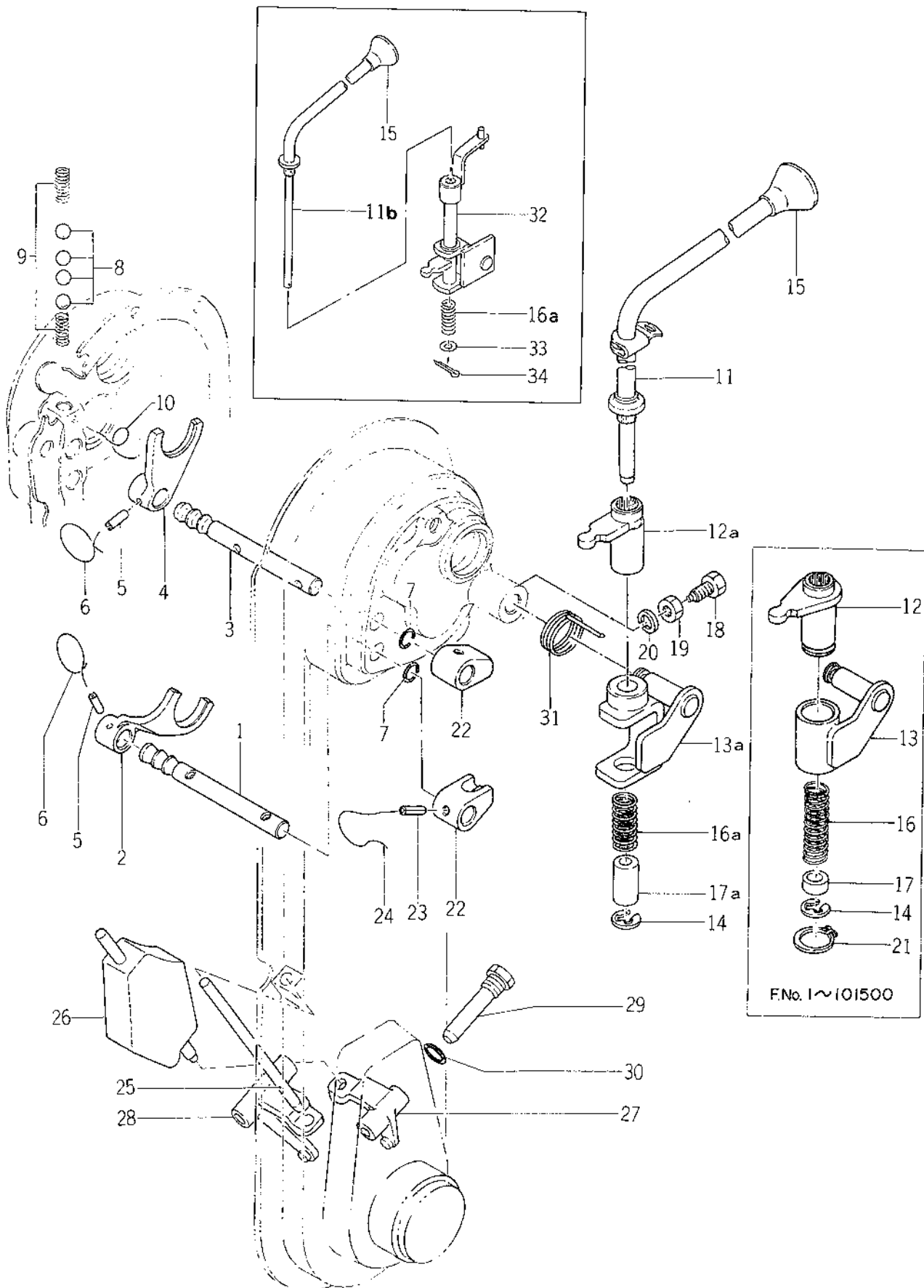
Fig. 10 SHIFTER Fourchettes
