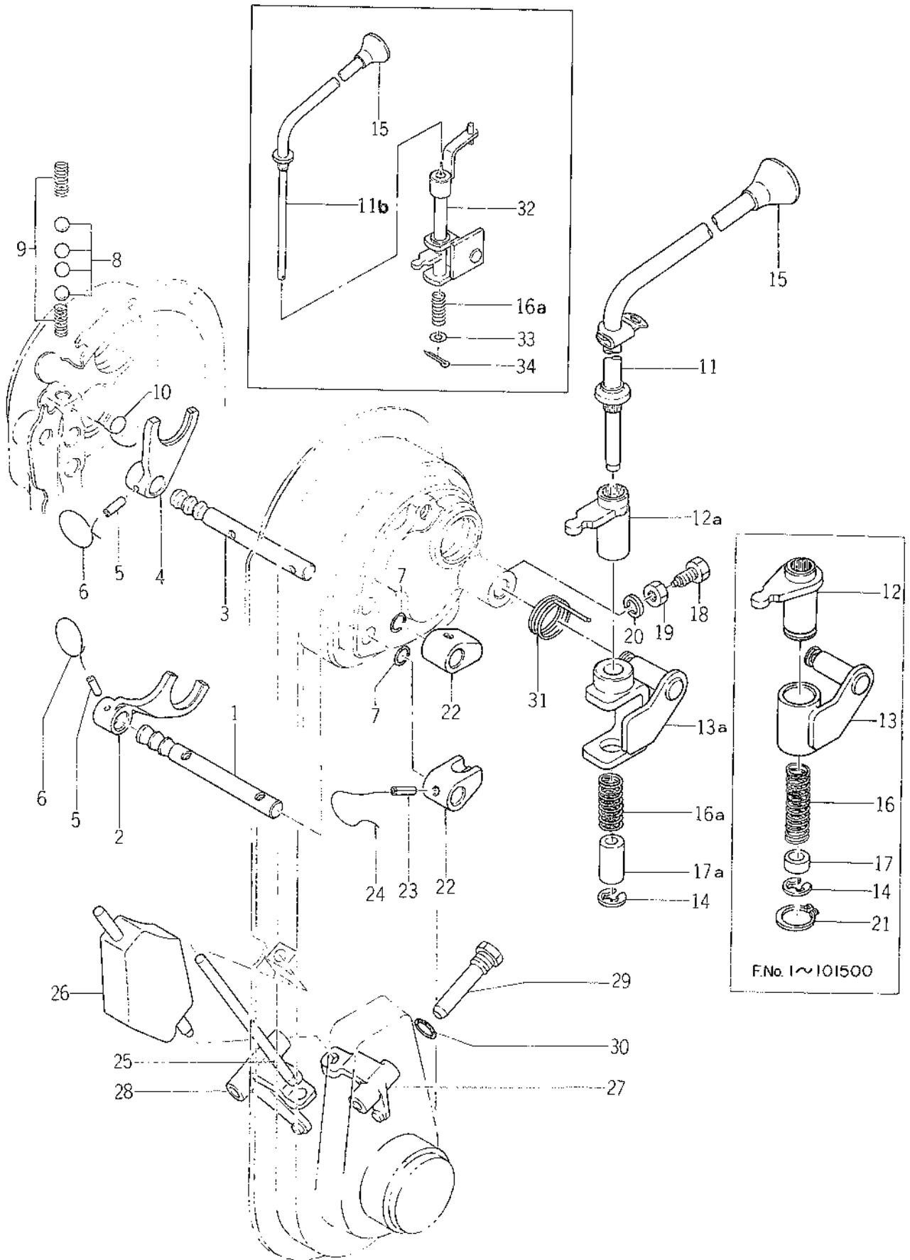
Fig. 10 SHIFTER Fourchettes
