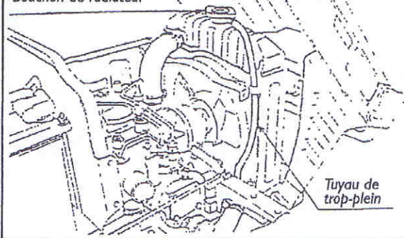
Bouchon de radiateur
